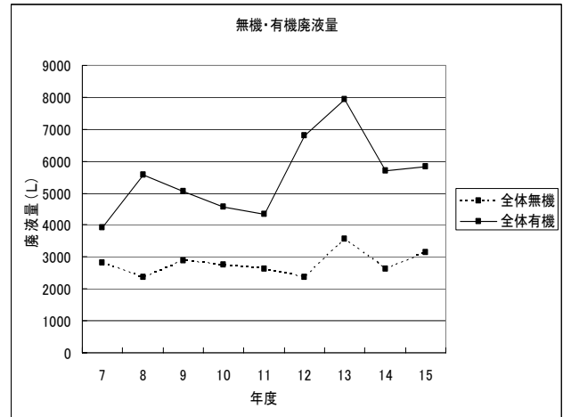
図3 全学部実験廃液量の経年変化
