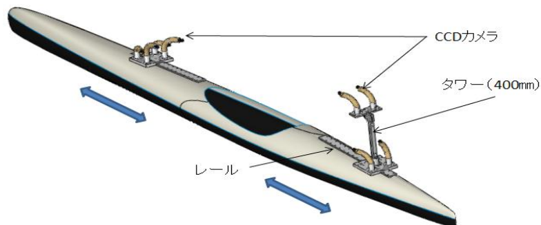
図 1 カヌー選手の動作解析装置 (3D CAD データ)
