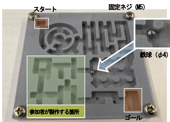
図4 迷路盤
