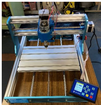
図6 小型 CNC フライス盤
